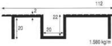
9715 Alt Kızak
