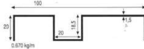
6126 Üst Kızak
