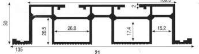
6655 3'lü Ray
