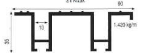
2132 2'lü Kızak
