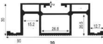
8412 2'lü Ray
