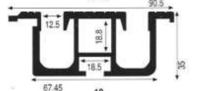
3425 2'lü Ray
