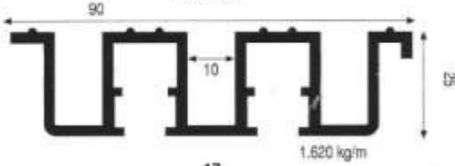
2131 3'lü Kızak
